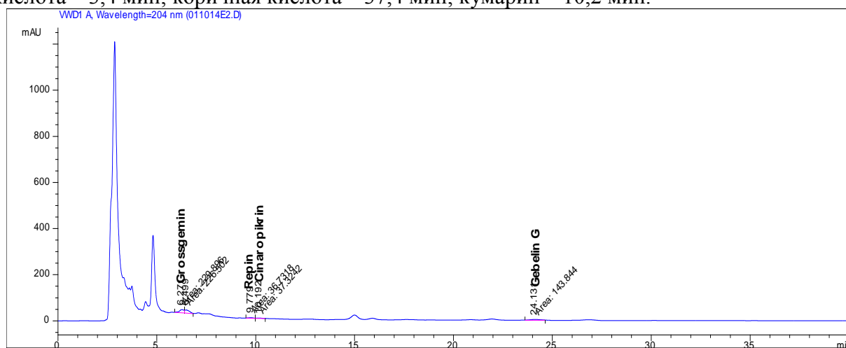
Рисунок 1 – Хроматограмма сесквитерпеновых лактонов спиртового экстракта соссюреи обернутой
