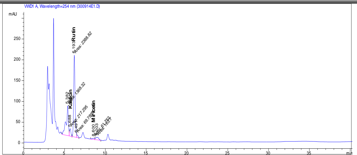
Рисунок 2 – Хроматограмма флавоноидов спиртового экстракта сосюреи обвернутой
