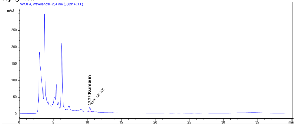
Рисунок 3 – Хроматограмма кумарина спиртового экстракта сосюреи обвернутой
