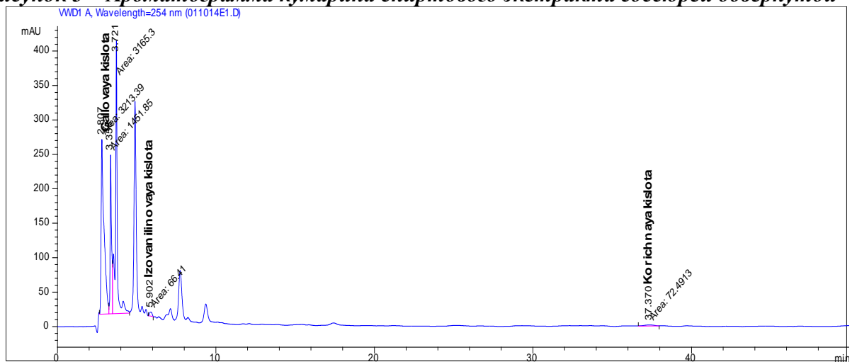
Рисунок 4 – Хроматограмма фенолокислот спиртового экстракта сосюреи обвернутой
