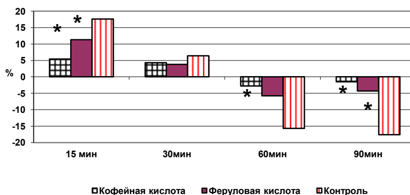
Рисунок 1. - Влияние кофейной и феруловой кислот на динамику постшемических цереброваскулярных феноменов
