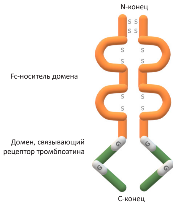
Рисунок 1 – Химическая структура ромиплостима
